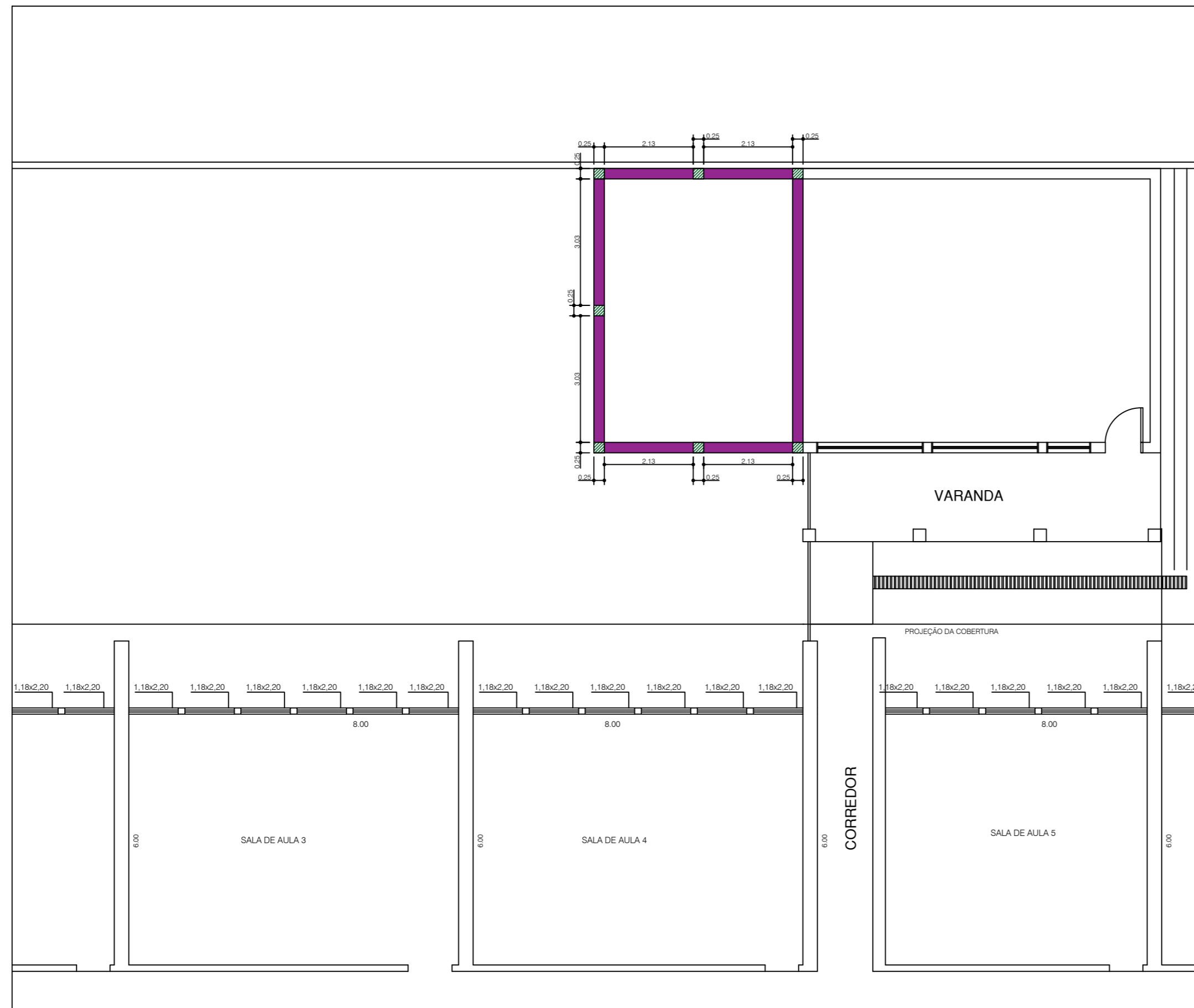
PLANTA SALAS - PILARES E VIGAS SUPERIORES
